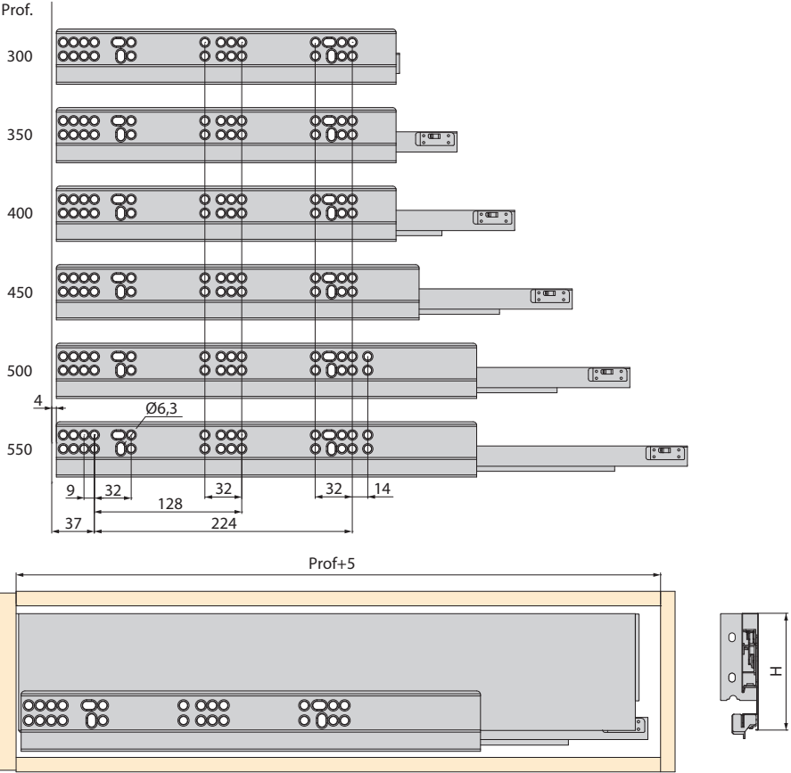
Panel dimensions / Dimensioni dei pannelli Dimensiones de paneles / Dimensions des panneaux Dimensões dos painéis / Wymiary panelu
